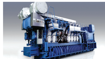
2000 09 선박용 디젤엔진 독자모델 · 현대힘센 · 엔진 개발
